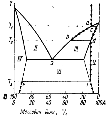
Рис. 32. Диаграмма плавкости бинарной системы с ограниченной растворимостью компонентов в твердом состоянии
