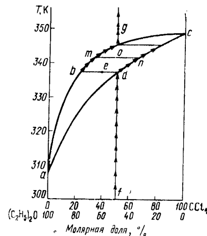
Рис. 25. Диаграмма кипения системы (\text{C}_2\text{H}_5)_2\text{O}-\text{CCl}_4 при 1,0133 \cdot 10^5 Па
