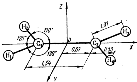
Рис. 47. Определение координат центра тяжести молекулы CH_2=CH_2
