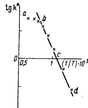
Рис. 50. Зависимость \lg k от 1/T для реакции окисления угля кислородом воздуха
