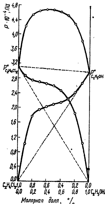
Рис. 22. Зависимость парциальных и общего давления пара от состава системы \text{C}_2\text{H}_5\text{Cl}-\text{C}_2\text{H}_5\text{OH} при 313 К
