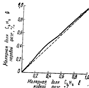
Рис. 24. Зависимость состава пара от состава жидкой фазы для системы \text{C}_6\text{H}_6-\text{C}_2\text{H}_4\text{Cl}_2 при 313 К
