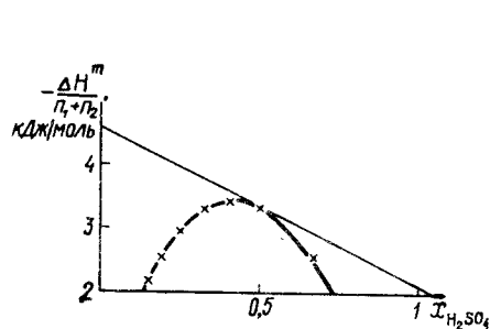
Рис. 18. Зависимость теплоты растворения серной кислоты в воде от молярной доли раствора
