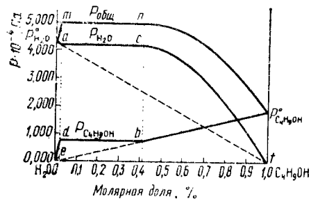
Рис. 28. Зависимость парциальных и общего давления от состава системы H_2O-C_6H_5OH с ограниченной растворимостью при 350 К
