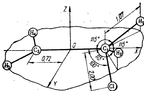
Рис. 48. Предполагаемая структура активированного комплекса
