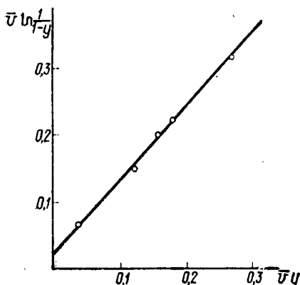
Рис. 52. Зависимость \bar{v} \ln от \bar{v} y для реакции каталитической дегидратации этилового спирта
