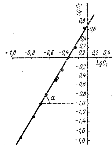
Рис. 20. Зависимость логарифма концентрации c_2 бензольного раствора салициловой кислоты от логарифма концентрации c_1 салициловой кислоты в воде
