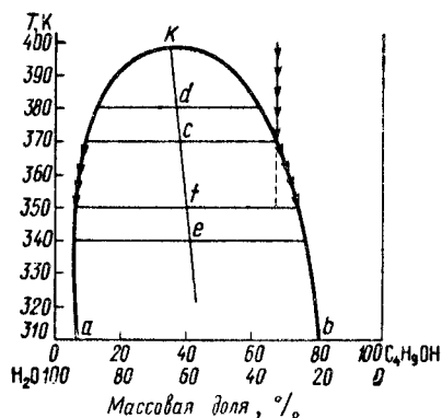
Рис. 27. Диаграмма фазового состояния системы \text{H}_2\text{O} - \text{C}_4\text{H}_9\text{OH} с ограниченной растворимостью компонентов
