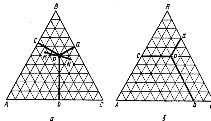
Рис. 37. Изображение составов трехкомпонентной системы методом Гиббса (а) и методом Розебума (б)
