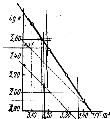
Рис. 45. Зависимость \lg k от 1/T для реакции C_6H_5N + CH_3I \rightarrow [C_6H_5NCH_3]^+ + I^-
