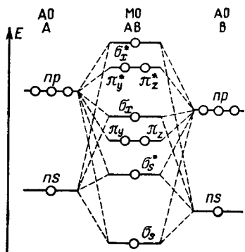
Рис. 2. Относительное расположение молекулярных орбиталей по энергии гетероядерных двухатомных молекул
