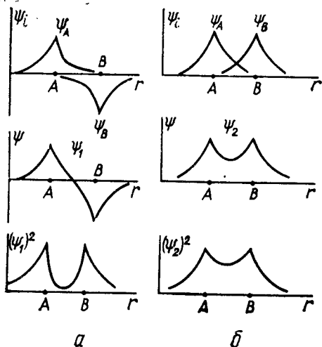
Рис. 3. Разрыхляющая (а) и связывающая (б) ионные функции гомоядерной двухатомной молекулы
