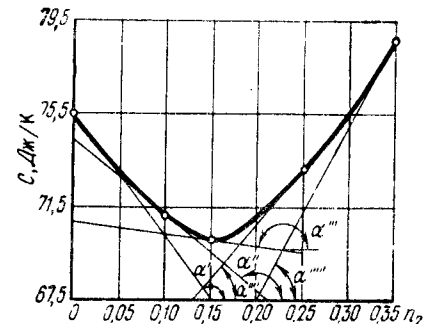
Рис. 19. Зависимость теплоемкости водного раствора HCl от содержания HCl в растворе
