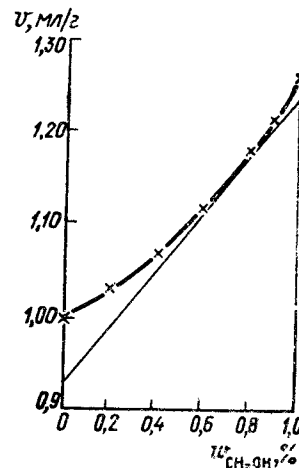
Рис. 16. Зависимость объема раствора \text{CH}_3\text{OH} в \text{H}_2\text{O} от молярной доли
