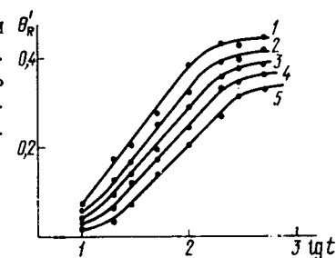
Рис. 56. Кинетические кривые адсорбции малеиновой кислоты при различных температурах; °С; 1 — 60; 2 — 50; 3 — 40; 4 — 30; 5 — 20
