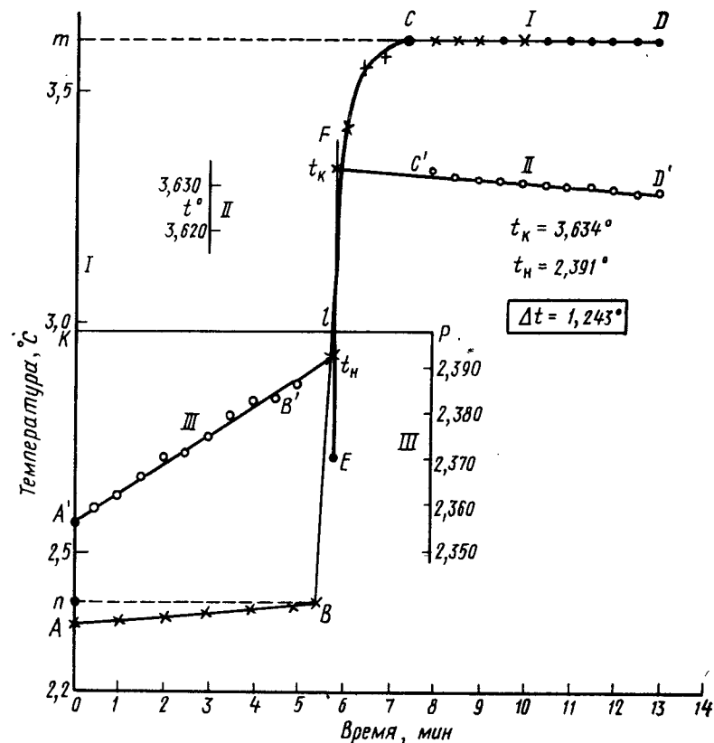
Рис. 10. Определение изменения температуры в ходе калориметрического опыта при больших тепловых эффектах
