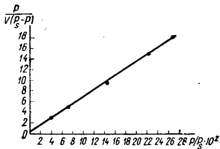
Рис. 41. Зависимость P/[V(P_s - P)] от P/P_s
