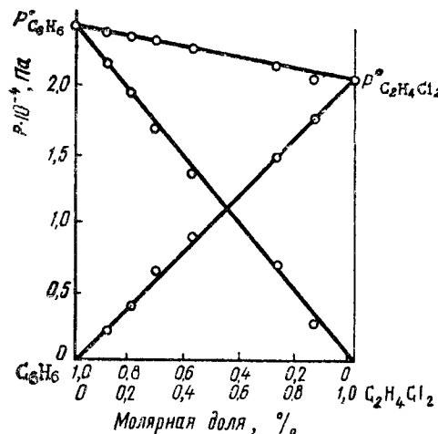
Рис. 21. Зависимость парциальных и общего давления пара от состава системы C_6H_6-C_2H_4Cl_2 при 313 К
