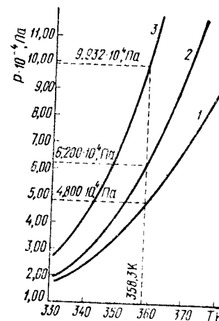
Рис. 29. Зависимость давления насыщенного пара от температуры для C_6H_5CH_3 (1), H_2O (2) и системы H_2O-C_6H_5CH_3 (3)
