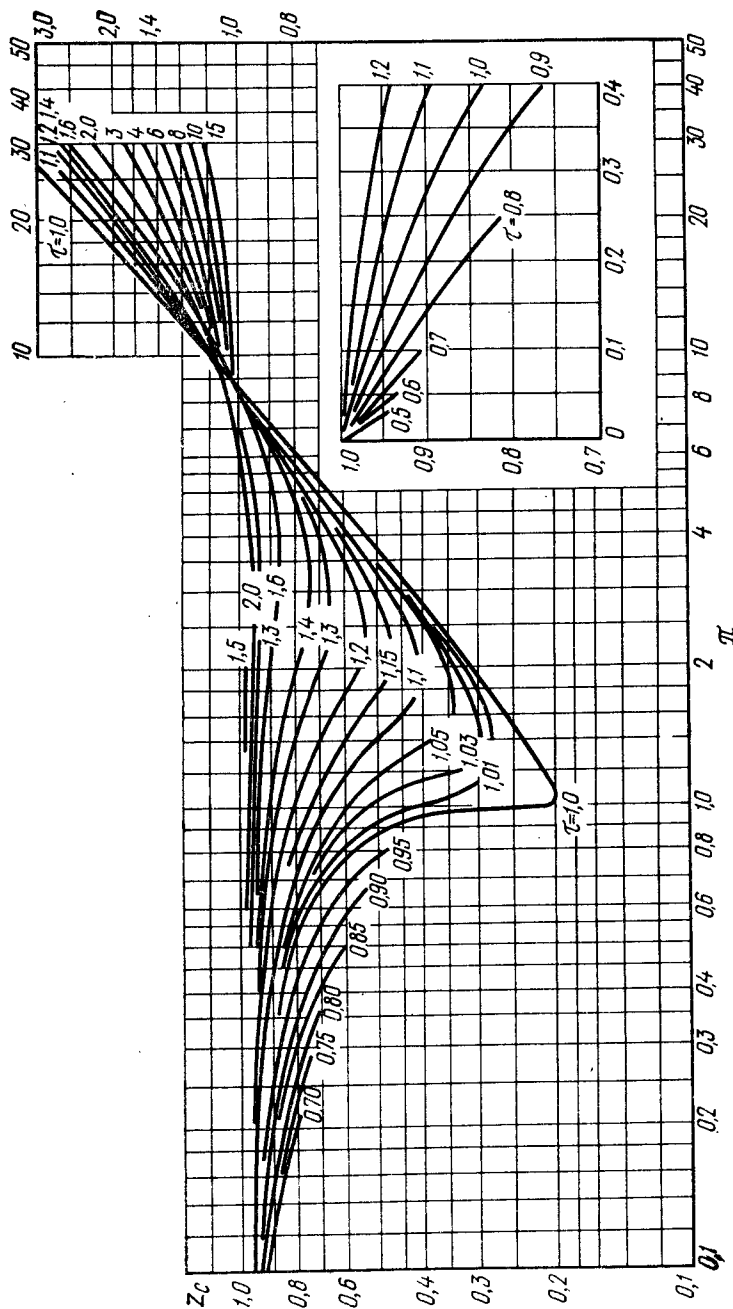
Рис. 14. Зависимость коэффициента сжимаемости z от приведенного давления p и приведенной температуры T
