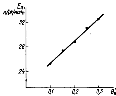
Рис. 58. Изменение энергии активации от степени заполнения поверхности
