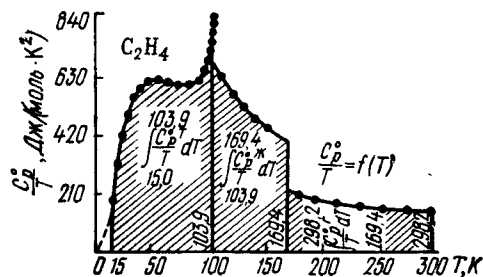
Рис. 11. Зависимость C_p^0/T от температуры для этилена
