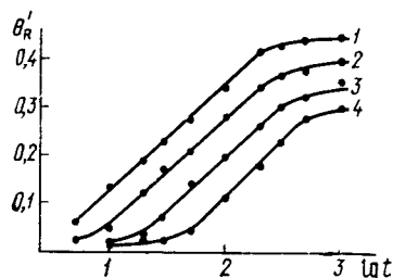
Рис. 54. Зависимость степени заполнения поверхности малеиновой кислотой различной концентрации от времени адсорбции, моль/л:
