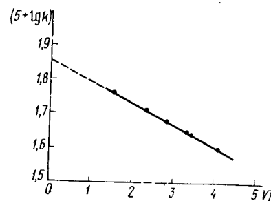
Рис. 53. Зависимость \lg k от \sqrt{I} для реакции \text{Co}(\text{NH}_3)_5\text{NO}_2^{2+} + \text{OH}^- \rightarrow \text{Co}(\text{NH}_3)_5\text{OH}^{2+} + \text{NO}_2^-
