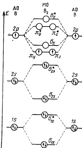
Рис. 4. Относительное расположение электронных уровней молекулы B_2 и заполнение АО и МО электронами
