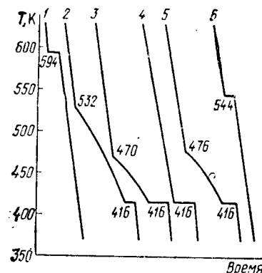
Рис. 35. Кривые охлаждения системы Cd—Bi: 1 — 0% Bi; 2 — 20% Bi; 3 — 40% Bi; 4 — 60% Bi; 5 — 80% Bi; 6 — 100% Bi
